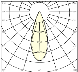
Curva fotometrica 36° 2700K 1140lm
