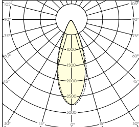
Curva fotometrica 36° 4000K 1270lm
