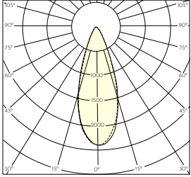
Curva fotometrica 36° 3000K 1170lm
