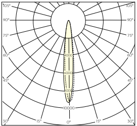
Curva fotometrica 12° 2700 K | 3000 K | 4000 K 970 lm | 1,140 lm | 1,140 lm
