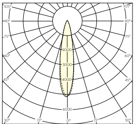
Curva fotometrica 24° 3000K 1170lm
