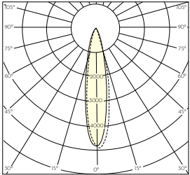
Curva fotometrica 24° 2700K 1140lm
