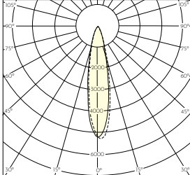
Curva fotometrica 24° 4000K 1270lm
